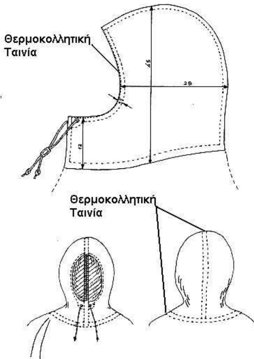
ΣΧΕΔΙΟ 3: ΛΕΠΤΟΜΕΡΕΙΕΣ ΚΟΥΚΟΥΛΑΣ ΑΤΟΜΙΚΟΥ ΑΔΙΑΒΡΟΧΟΥ (ΔΙΑΣΤΑΣΕΙΣ ΣΕ ΕΚΑΤΟΣΤΑ)
