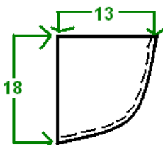
ΚΑΠΑΚΙ ΕΣΩΤΕΡΙΚΑ
