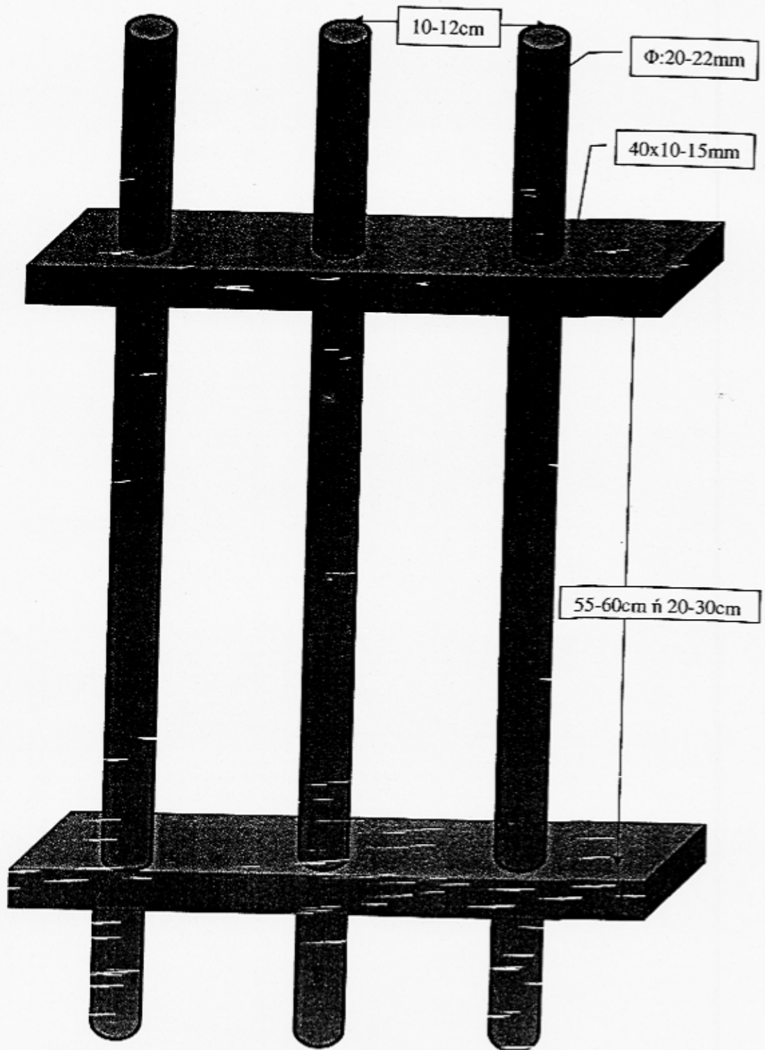
ΣΧΕΔΙΟ: Λεπτομέρεια Κατασκευής Κιγκλιδώματος
